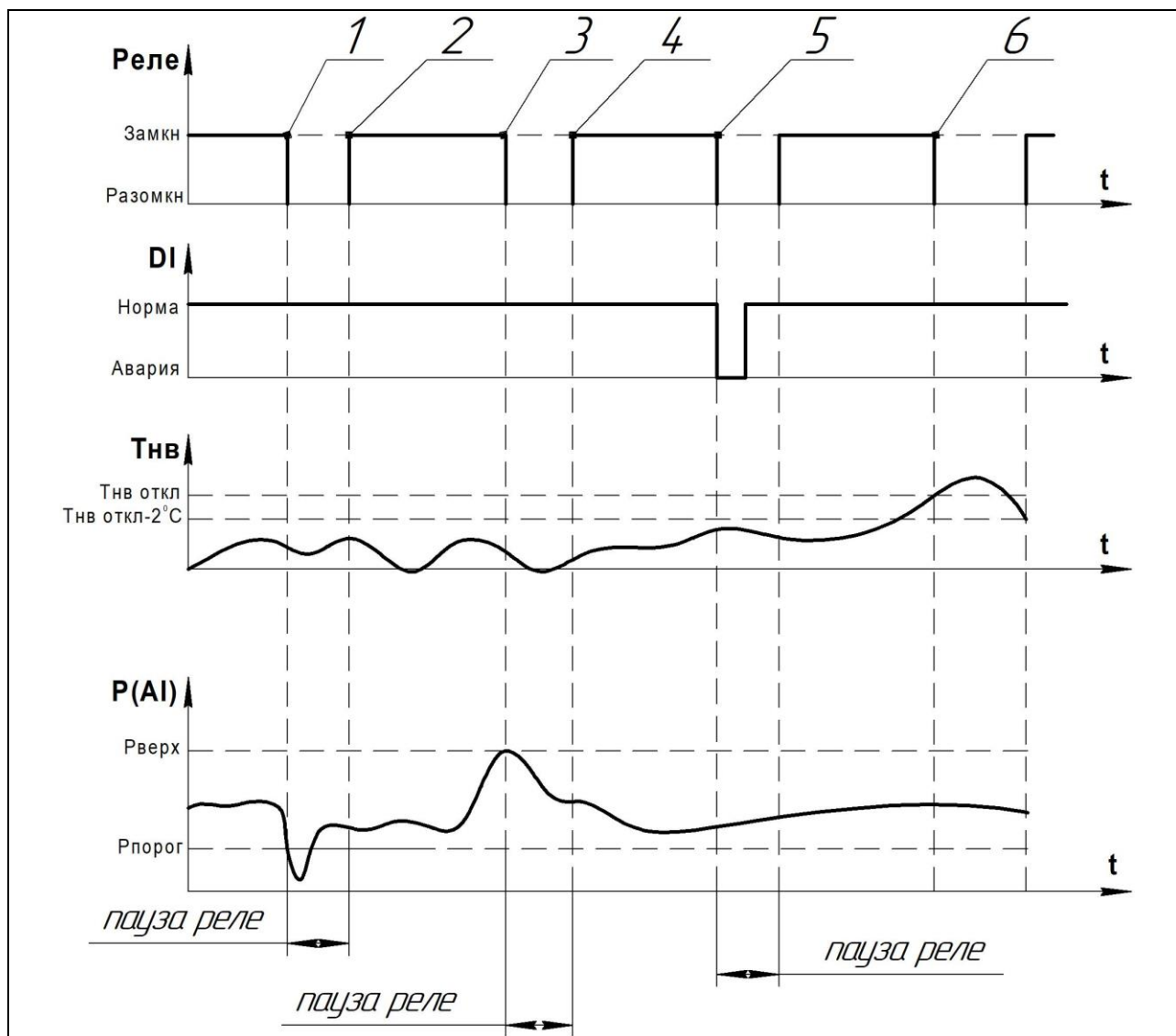
Рисунок 21 – Режим реле "ЦИРКУЛЯЦИЯ"
