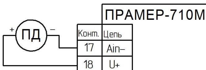
Рисунок 28,б – Подключение преобразователя давления (питание от встроенного источника постоянного тока)
