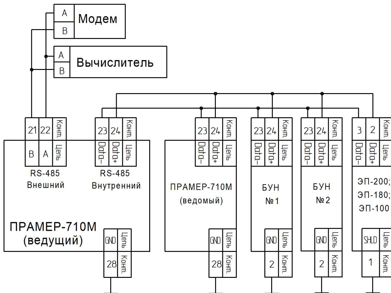
Рисунок 30 – Подключение интерфейса RS-485
