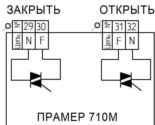
Рисунок 24 – Подключение ИМ
