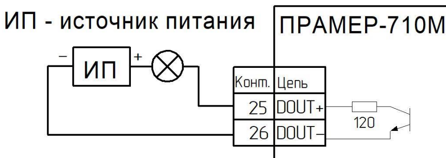
Рисунок 27 – Подключение к дискретному выходу контроллера.
