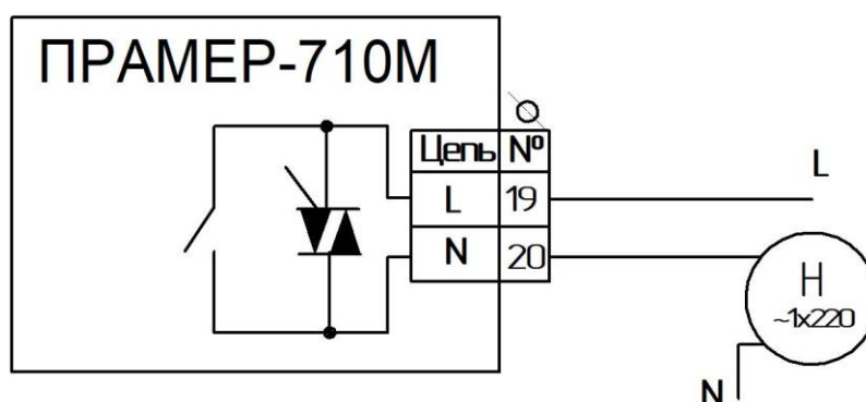
Рисунок 32 – Подключение к релейному выходу.
