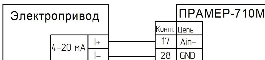
Рисунок 29 – Подключение датчика положения клапана.
