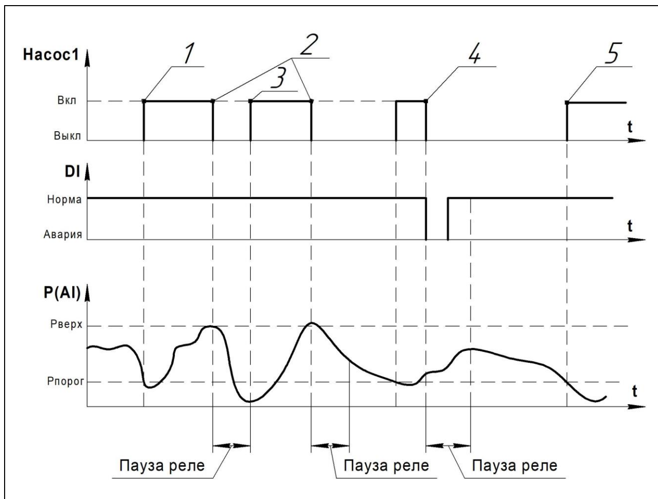
Рисунок 22 – Режим реле "ПОДПИТКА" :
