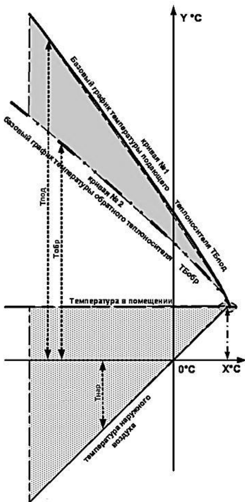
Рисунок 3 – Базовые графики теплоснабжения
