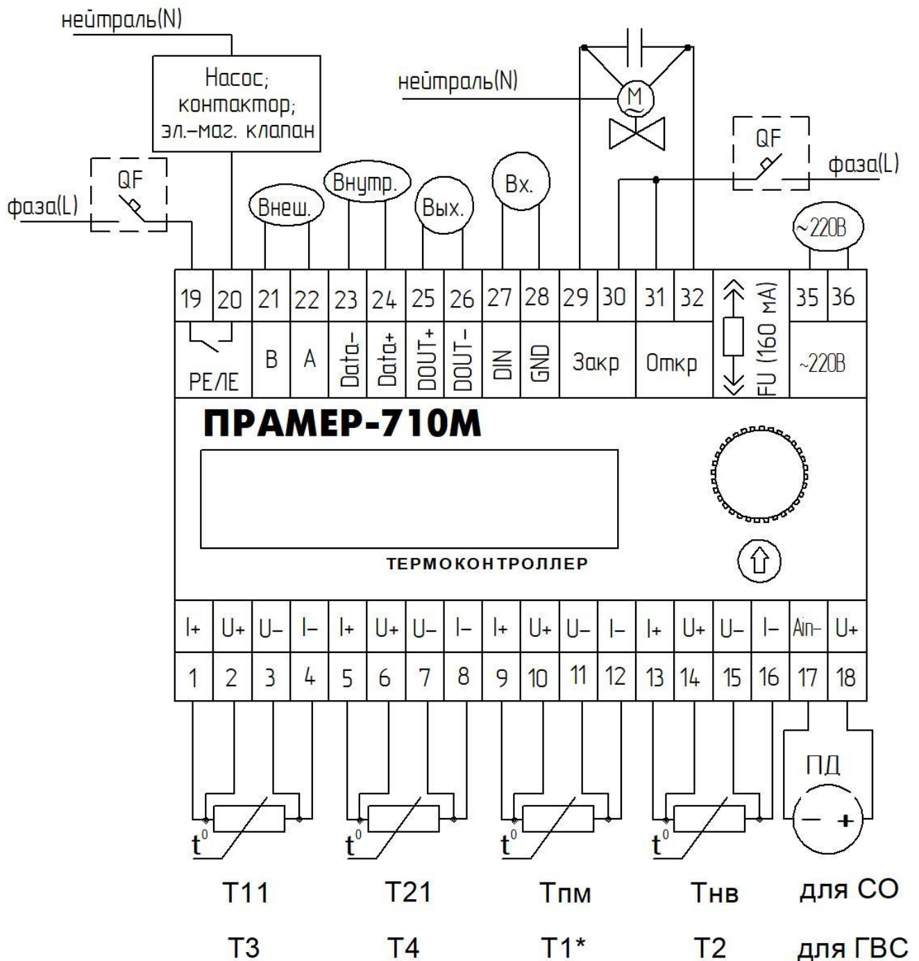
Рисунок Б.1 – Назначение клемм подключения внешних устройств
