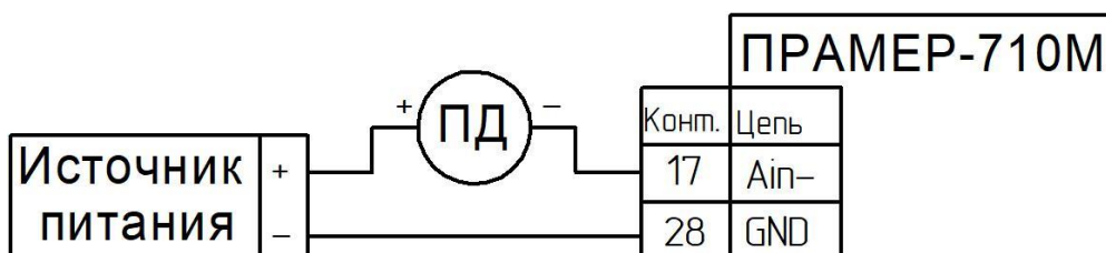
Рисунок 28,а – Подключение преобразователя давления (питание от внешнего источника)
