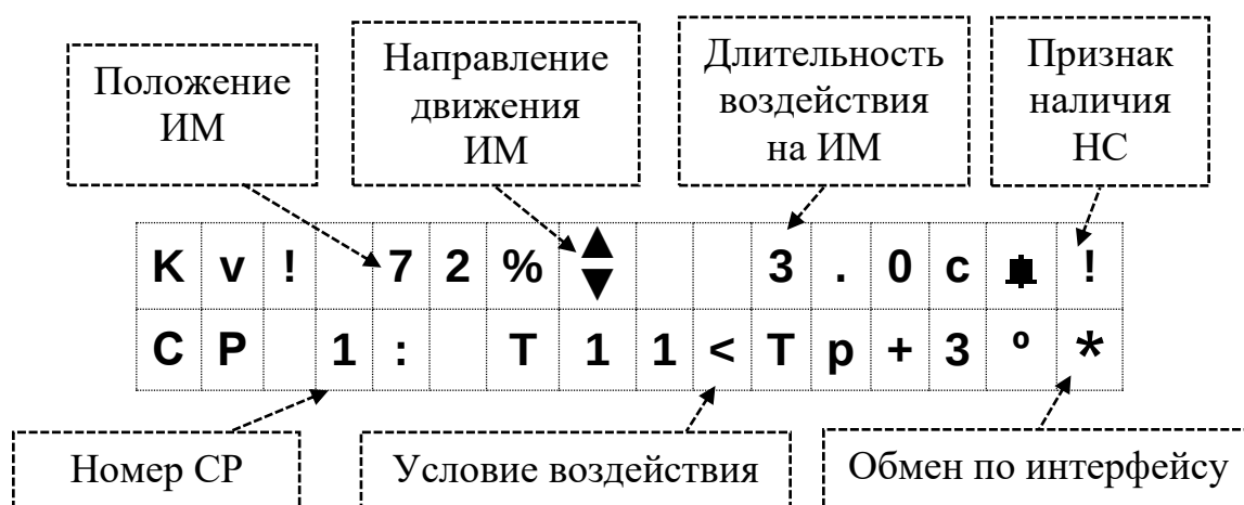
Рисунок 9 – Вид экрана индикатора в дежурном режиме
