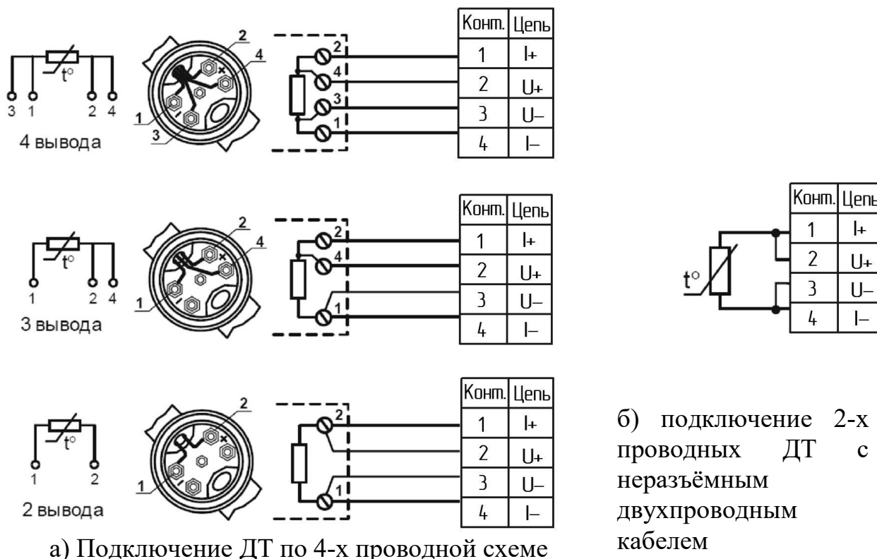
Рисунок 25 – Подключение ДТ
