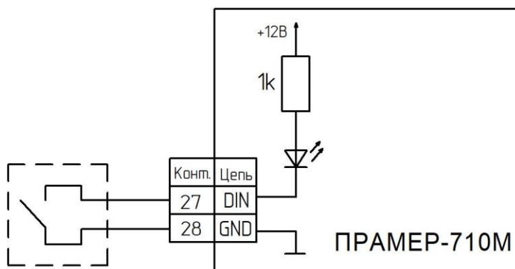
Рисунок 26 – Подключение к дискретному входу контроллера.
